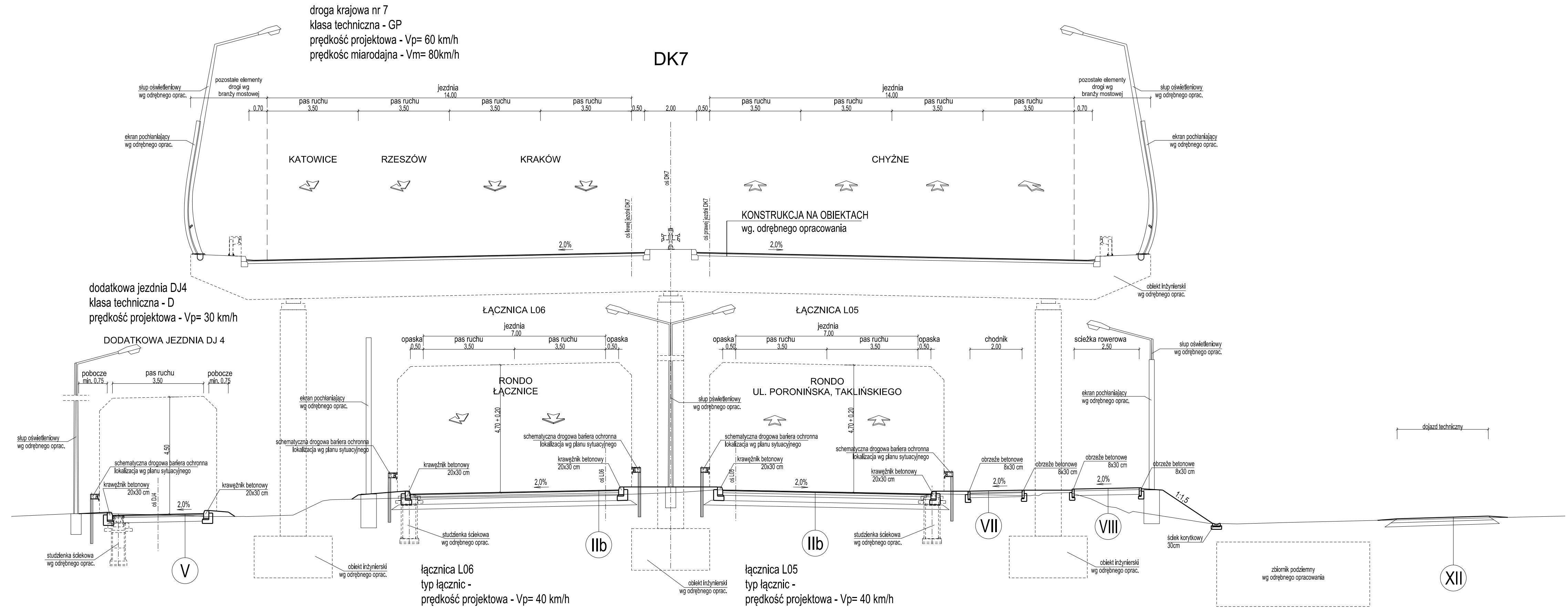
Przekrój charakterystyczny w km ok. 673+670 DK7
