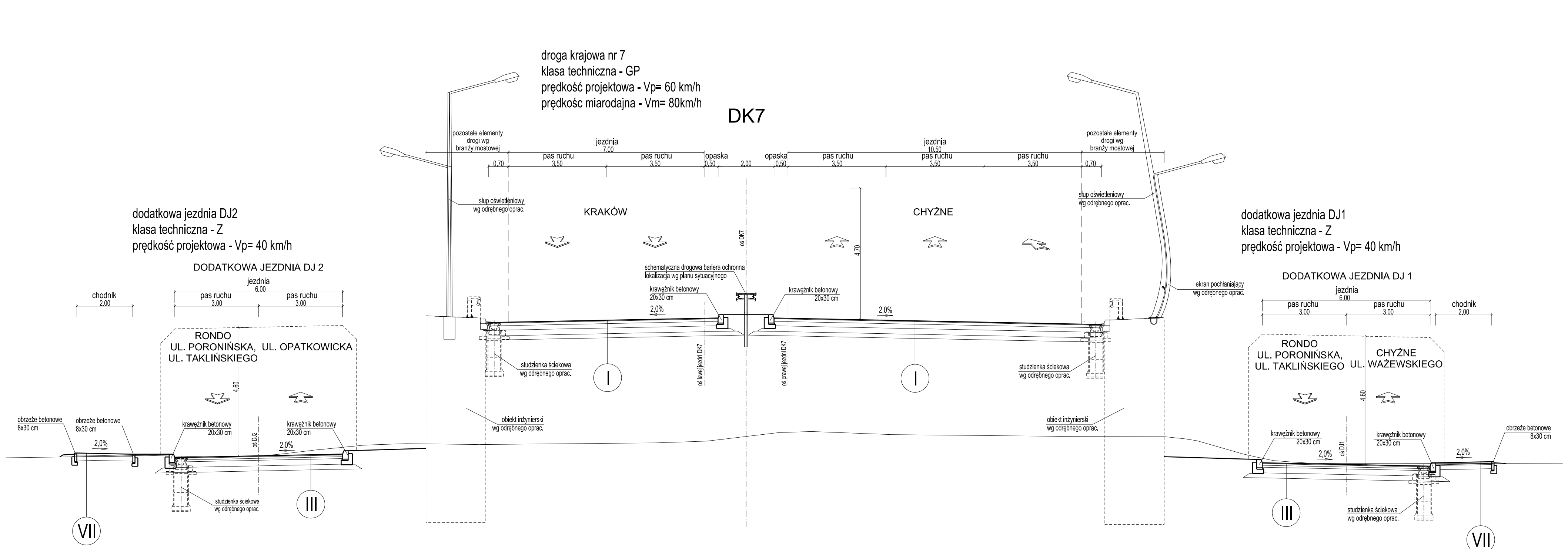
Przekrój charakterystyczny w km ok. 673+946 DK7
