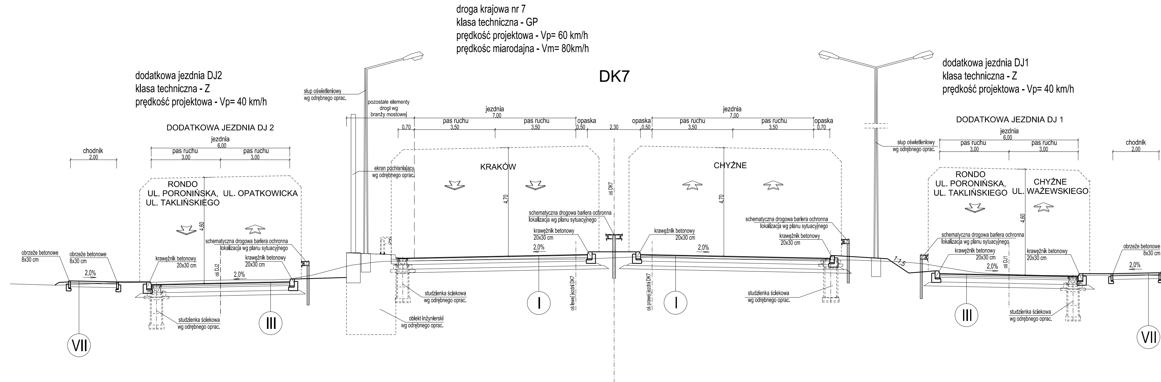
Przekrój charakterystyczny w km ok. 674+040 DK7
